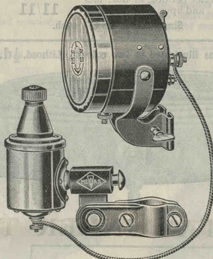
No. CIA/5. "MELAS" DYNAMO CYCLE LAMP SET. (F.)
