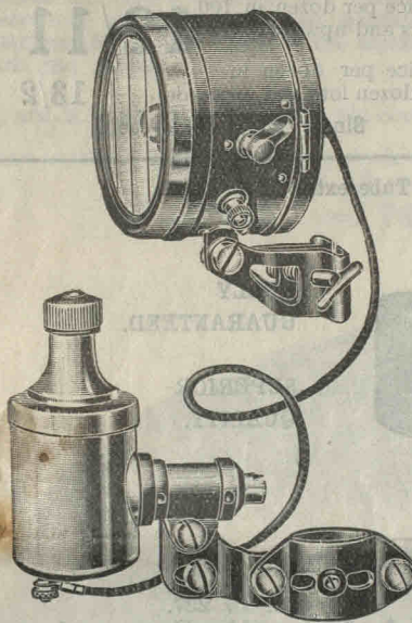
No. 61. "KIRMER" DYNAMO SET. (F.)
