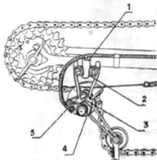
HURET "TOURISTE" DERAILLEUR GEAR (less Free Wheels)
