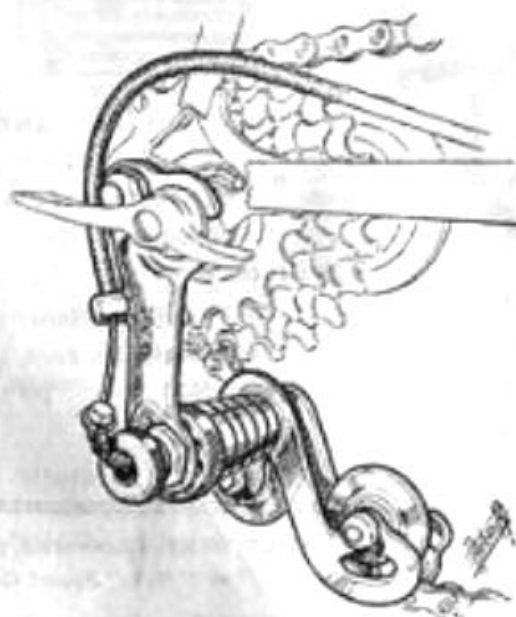
HURET "TOUR DE FRANCE" DERAILLEUR GEARS (less Free Wheels)
