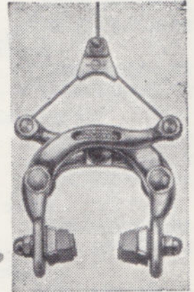
WEINMANN Vainqueur 999
