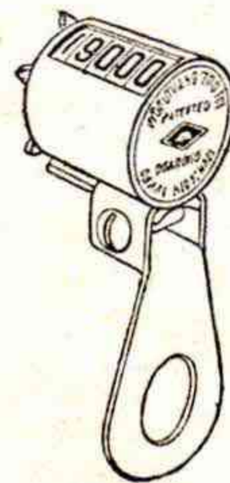
N:r 1967. Vägmätare för 28" hjul, förnicklad, registrerar väglängden intill 10,000 km. Pr st. 3: 50
