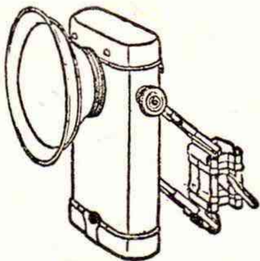
N:r 1185. Lykta, för velocipeder, av plåt, lackerad, storlek 65×105 mm., reflektor förnicklad 55 mm försedd med lens. Levereras med vanligt ficklampsbatteri och glödlampa. Kompl. .... Pr st. 2: 50
