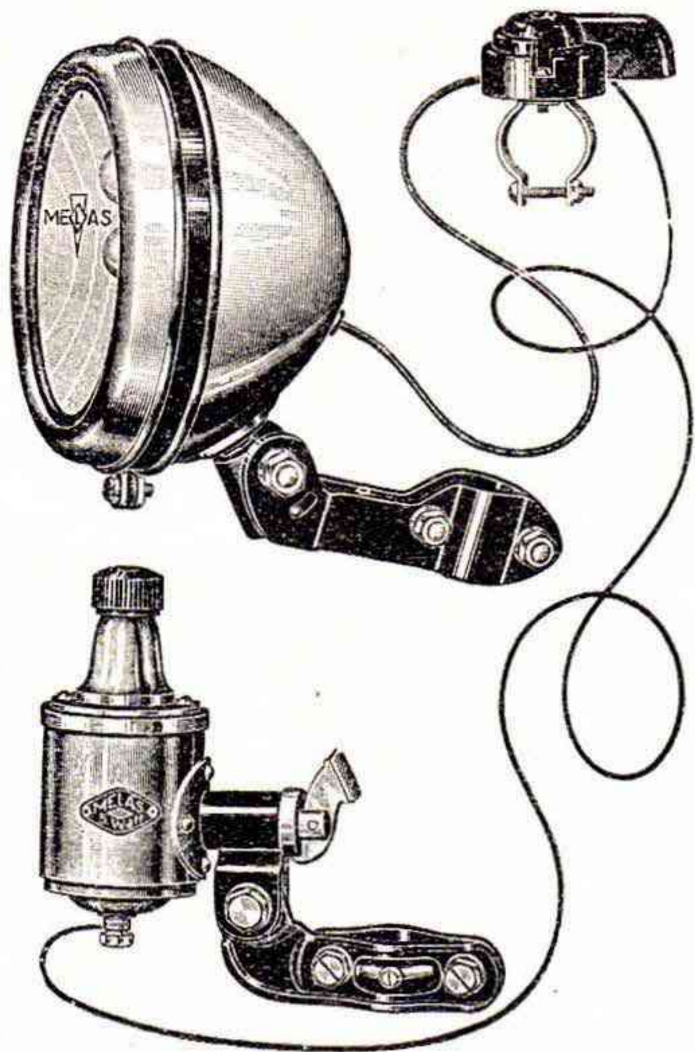
N:r 1169. Melas lyx, 6 volt, 5 watt, 2 lampor, hel- och halvljus samt strömbrytare att anbringa på styrstängen. Förkromad. Pr st. 21:—
